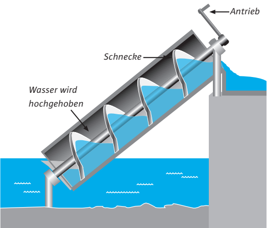
Darstellung der archimedischen Schraube
