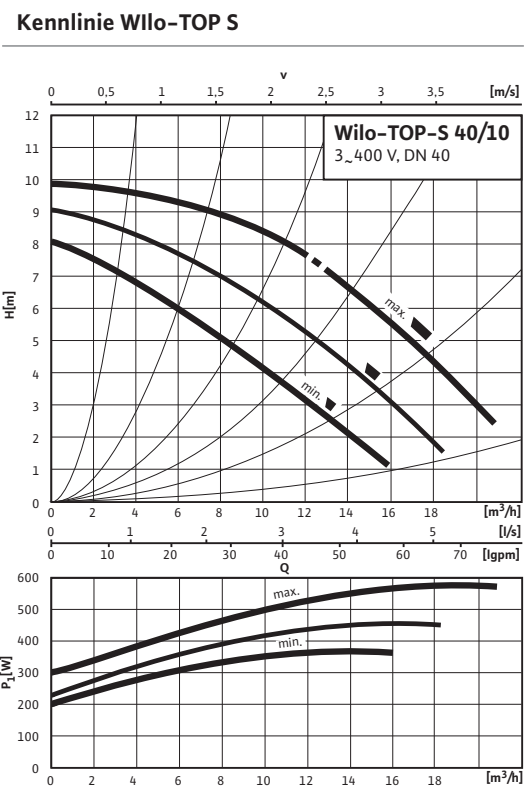
Nassläuferpumpe Wilo-TOP S mit 3 schaltbaren Drehzahlstufen
