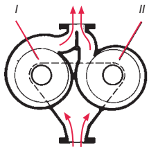
Beide Pumpen in Betrieb
