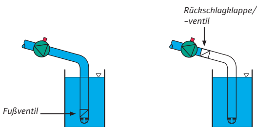
Installation mit Fußventil oder Rückschlagklappe/-ventil
