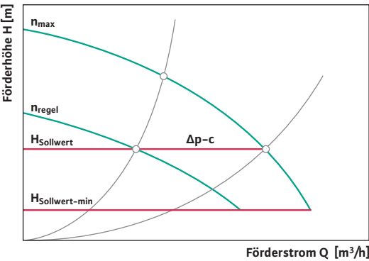
Differenzdruck konstant: \Delta p\text{-}c
