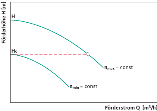
Betriebsart Handsteller
