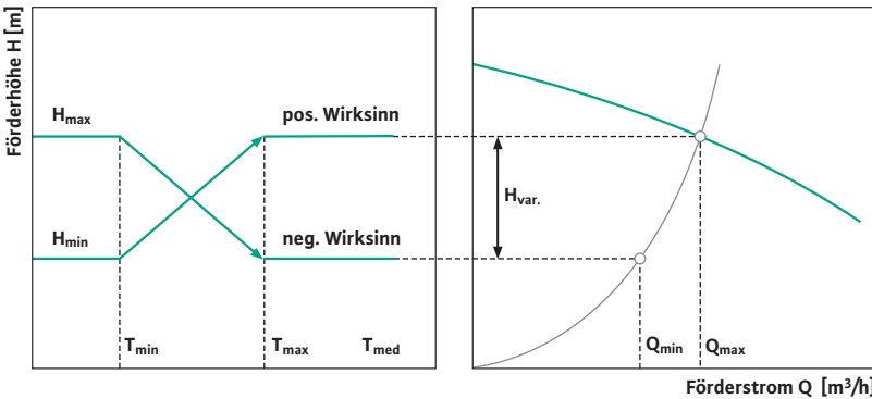
Temperaturgeführte Differenzdruckregelung: \Delta p\text{-}T in Abhängigkeit des sich daraus verändernden Förderstroms
