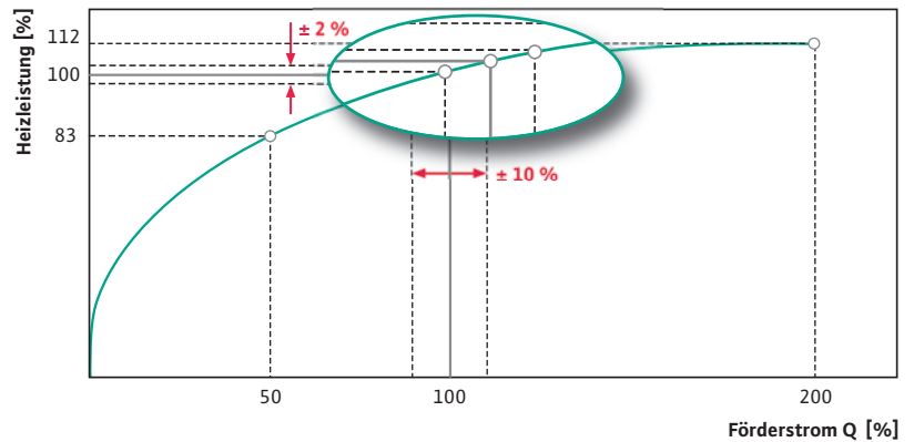
Heizkörper-Betriebsdiagramm
