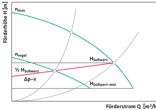
Differenzdruck variabel: \Delta p\text{-}v
