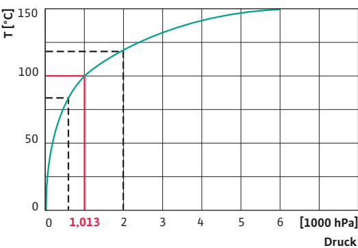
Siedepunkt des Wassers als Funktion des Drucks
